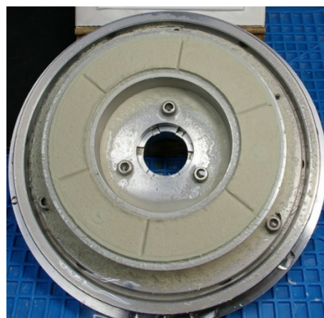
試験機に装填しドーナツ型にくり抜く
