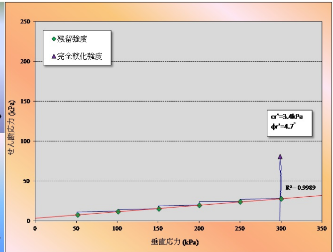
残留強度定数の決定
