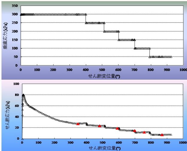
残留せん断強度の計測
