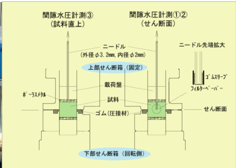
せん断箱付近の構造と間隙水圧の測定方法
